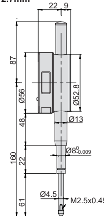
Range: 0-50.8mm
